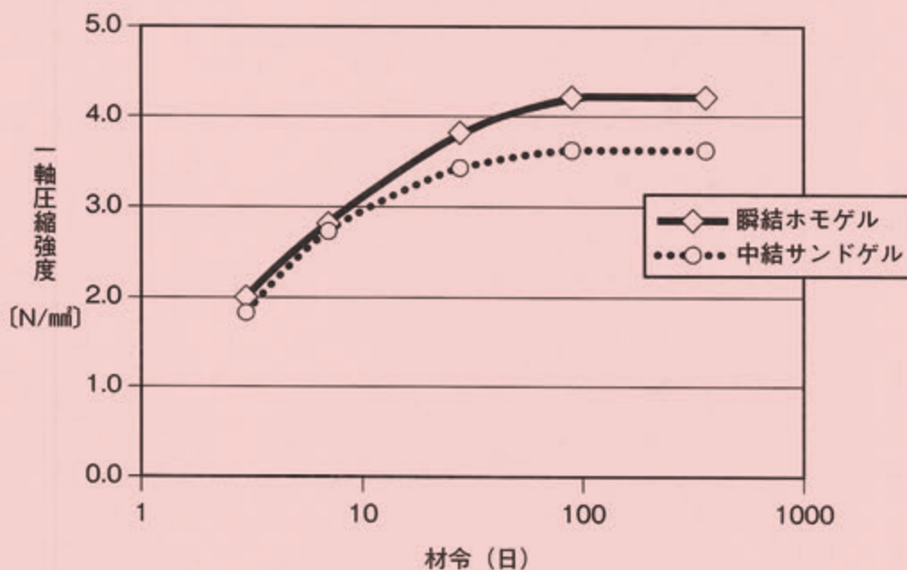
図3. 強度推移
