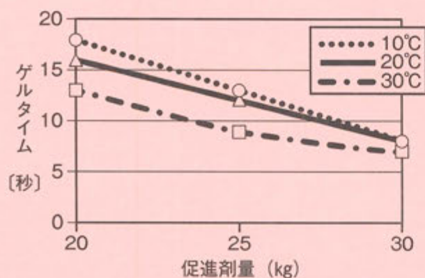
図1. 瞬結の促進剤量とゲルタイムの関係
